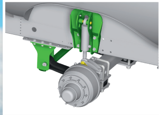
750/60R30.5 Trelleborg mit Reifendruckregelanlage
